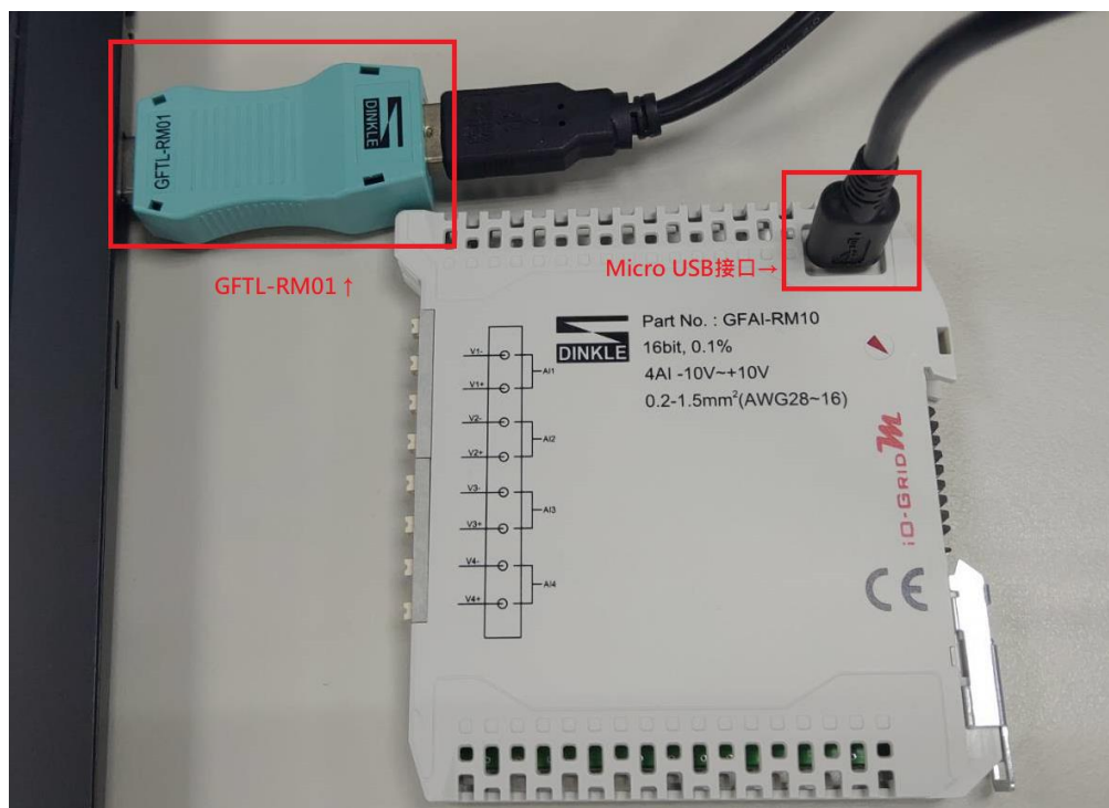
I/O 模組接線實體圖:
